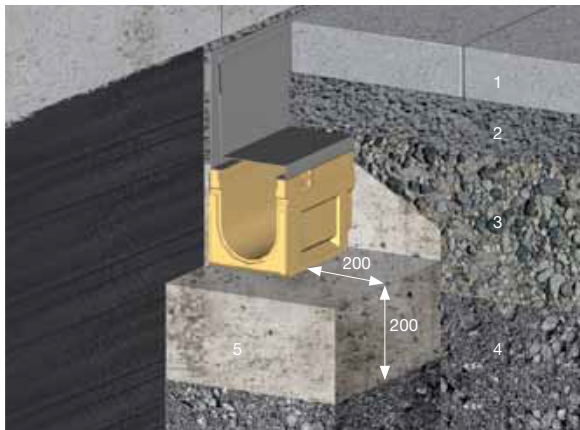
an Treppen- und Fassadenanschlüssen mit Plattenbelag
