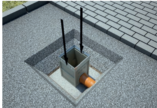
2. Hofeinlauf auf Betonbett setzen. Rohrleitung anschließen. Bei Anschluss eines Regenfallrohres, die Vorformung am Aufsatzkasten öffnen und Rohrstutzen einsetzen.
